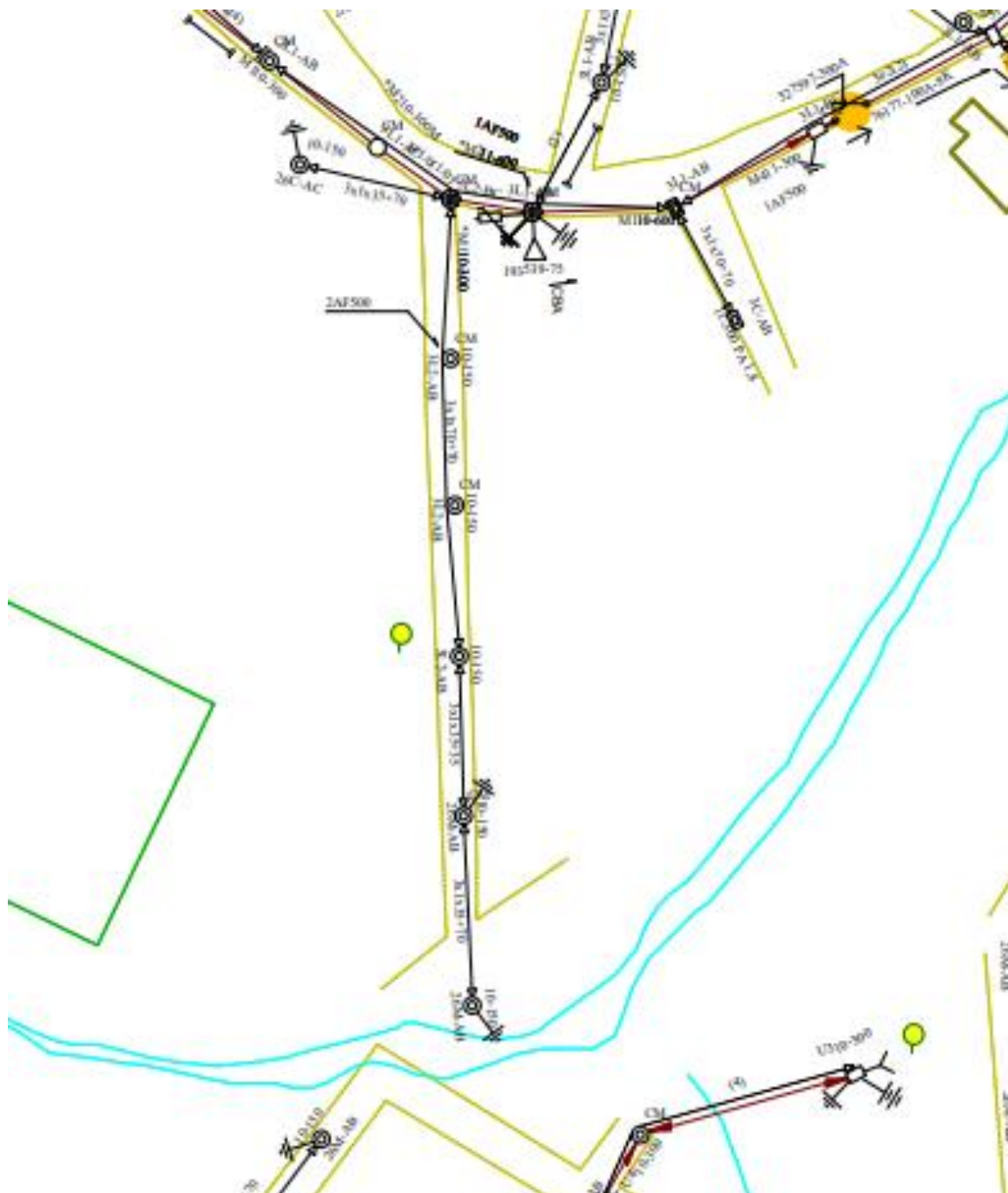
Figura 1: Vista do sistema Gemini da Cemig, indicando a existência de rede de posteamento com iluminação pública no local.
